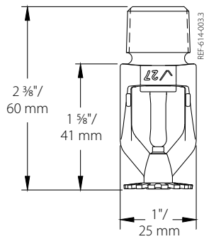
Colgante de respuesta estándar – V2707, V2708
