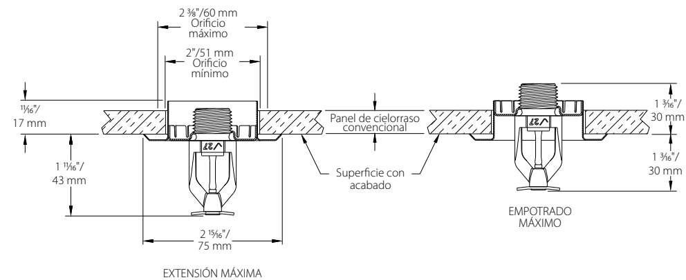
1/2" de ajuste, empotrado – V2707, V2708 (diagrama no está a escala)
