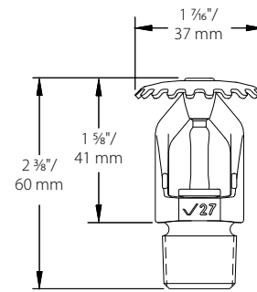
Vertical estándar – V2703, V2704
