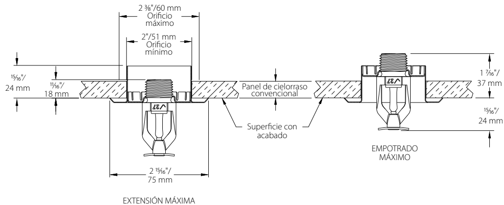
3/4" de ajuste, empotrado – V2707, V2708 (diagrama no está a escala)
